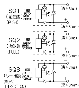
電気仕様 WIRING DIAGRAM
