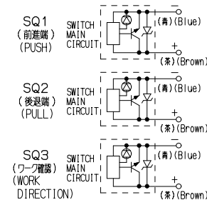
電気仕様 WIRING DIAGRAM
