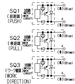
電気仕様 WIRING DIAGRAM
