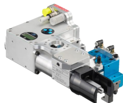
BR-AJC_E + 反力レバー + トルクスレンチ
