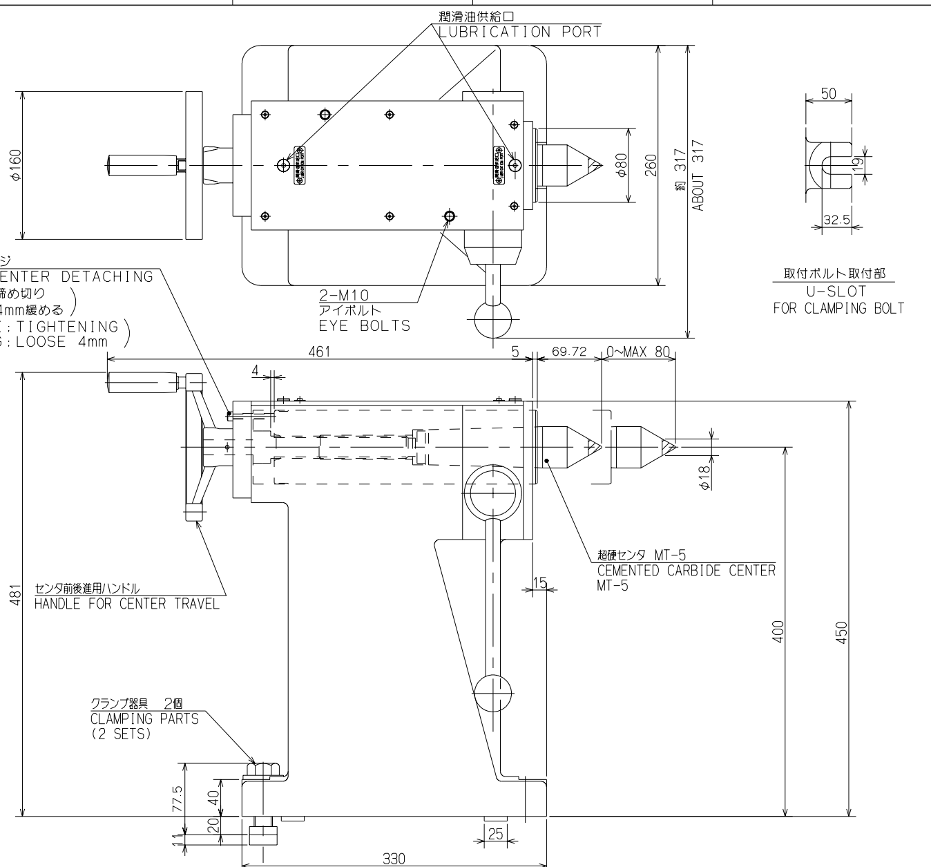
センタクランプレバー CENTER CLAMP LEVER
