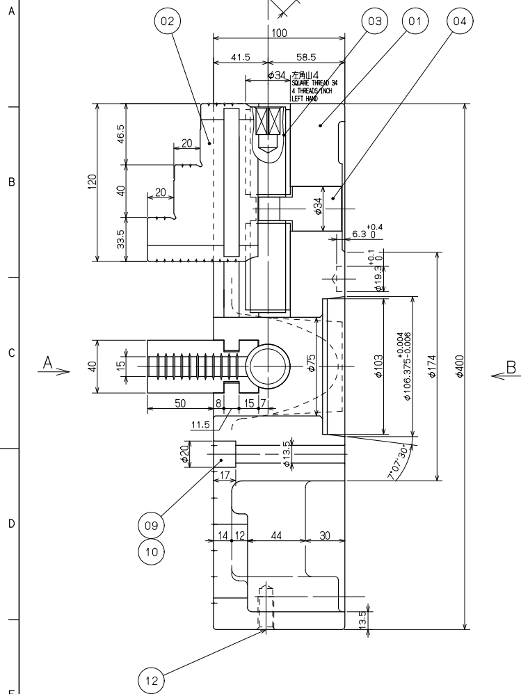
断面C-O-D SEC.C-O-D
