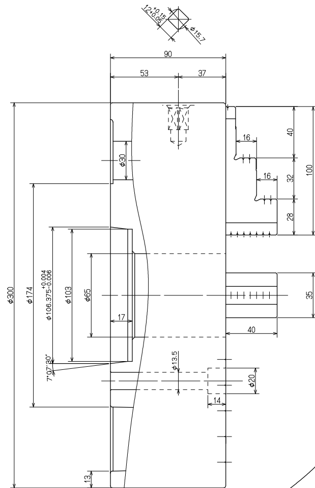
C-O-D 断面
