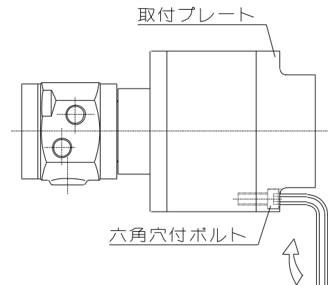
六角穴付ボルトの規定トルク
