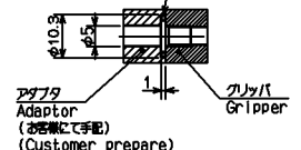
ベース配管接続 Detail of direct connecting
